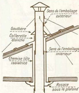
Traverse d'un grenier
