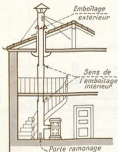
Installation dans une cage d'escalier
